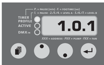
Fig. 6: Réglage du temps de pause (Pre-Runtime)
