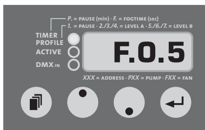
Fig. 11: Réglage de la durée d'émission de fumée (Fogtime) en sec. (1-99)
