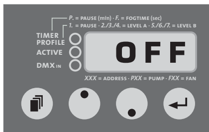
Fig. 5: L'arrêt de l'appareil.
